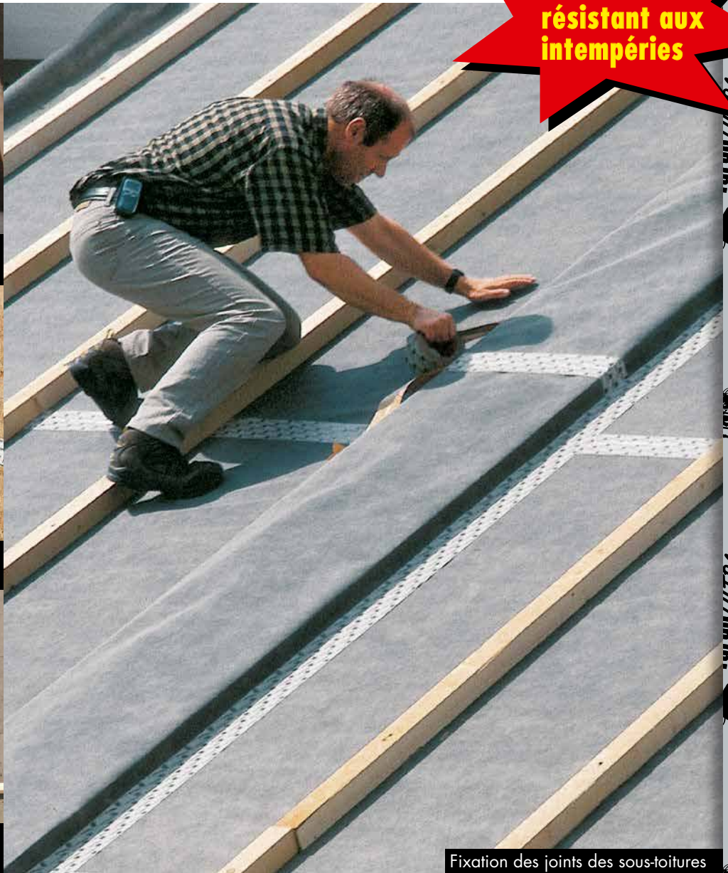
Raccords des sous-toitures et des coupe-vent
